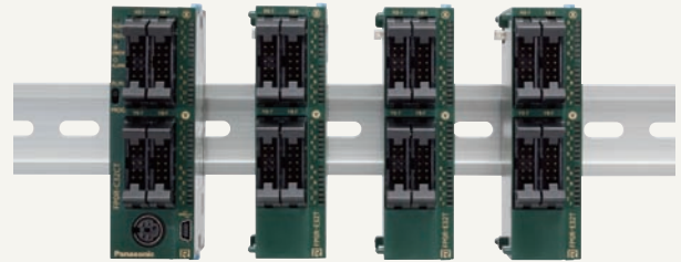
控制单元 ◀ 扩展单元 ◀ 扩展单元 ◀ 扩展单元 (最多可用3个扩展单元)
