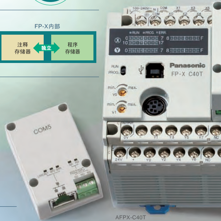
AFPX-C40T (安装扩展插件的状态下)
