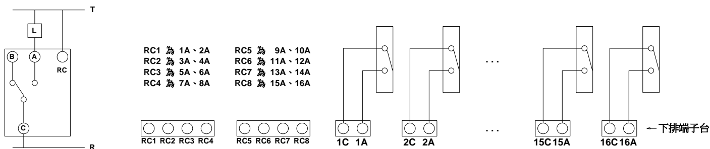
火花消除接線範例：
