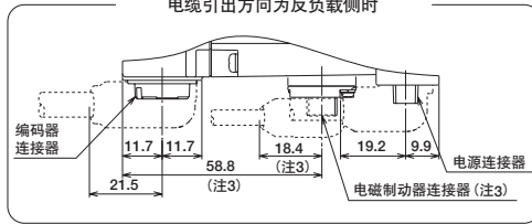
电缆引出方向为反负载侧时
