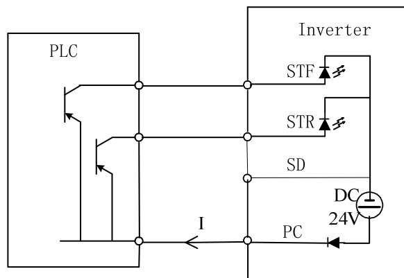
Source Input: 多功能控制端子與開發射極的PLC直接相連接
