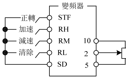
遠端控制設定的接線圖示例
