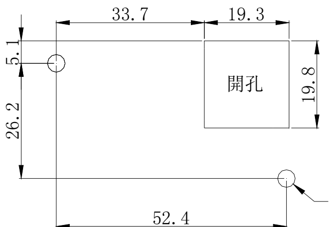
<螺絲安裝面板開孔尺寸圖>
