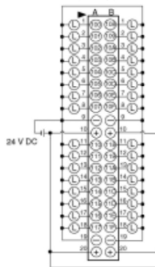
输出用连接器(PNP) (单元右侧)
