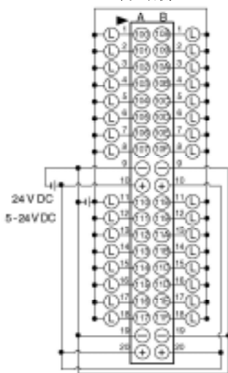
输出用连接器(NPN) (单元右侧)
