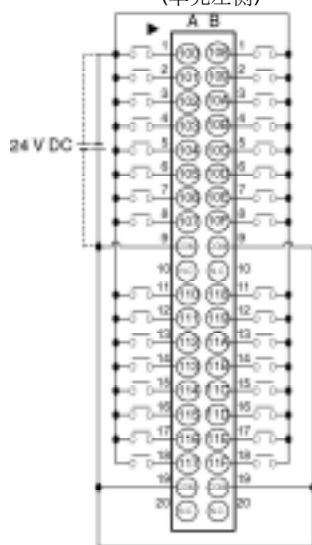
输入用连接器 (单元左侧)
