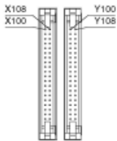
(连接器正面图)
