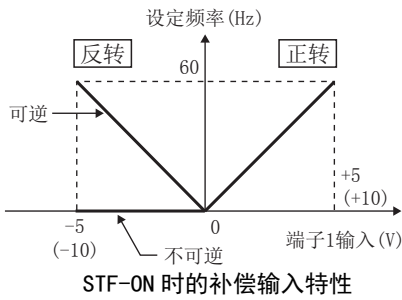
STF-ON 时的补偿输入特性
