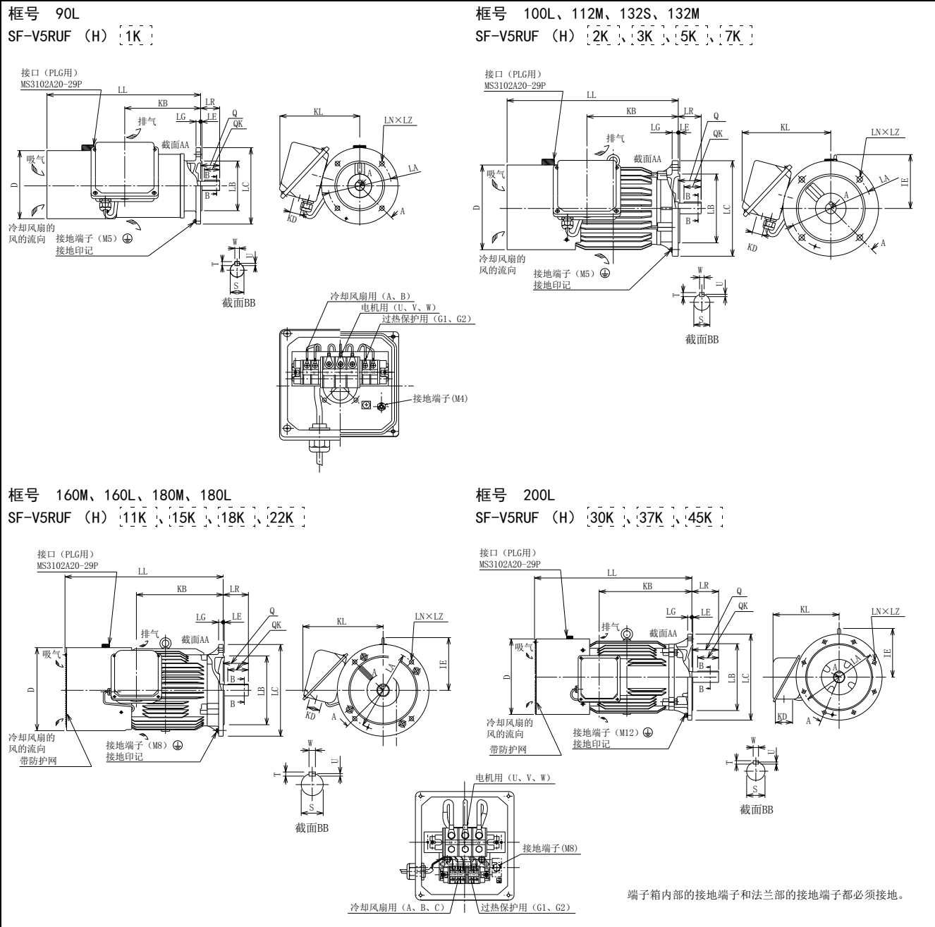
专用电机（SF-V5RU（H））外形尺寸图（法兰型）
