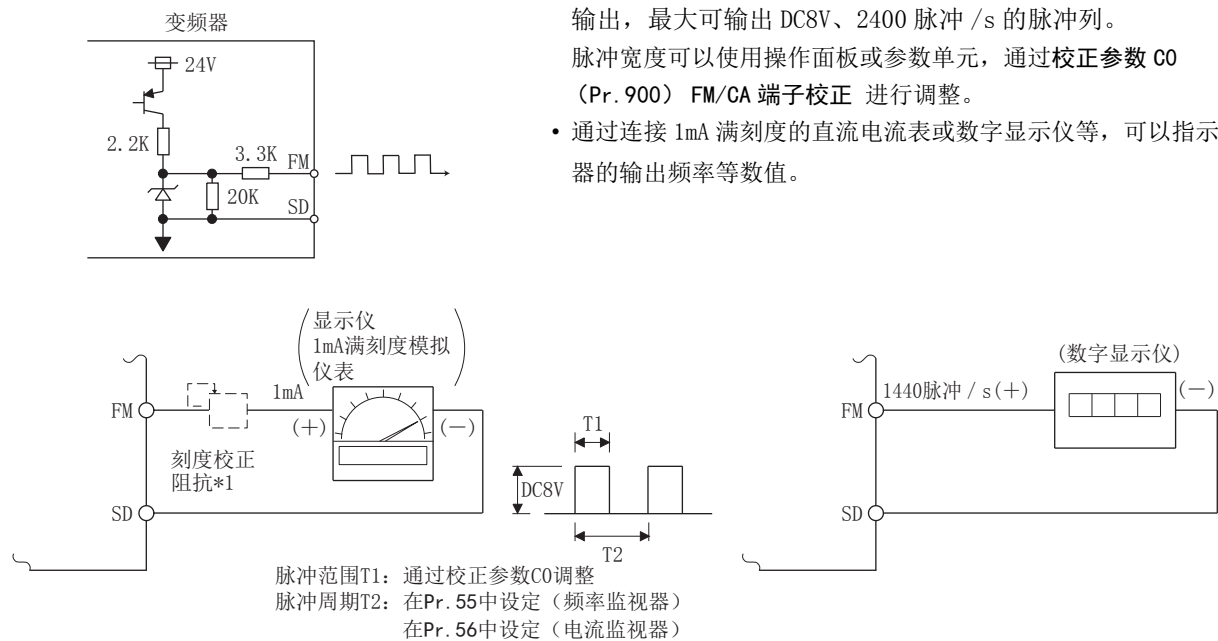
FM 输出回路
