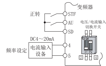
使用端子4 (DC4~20mA) 接线的示例
