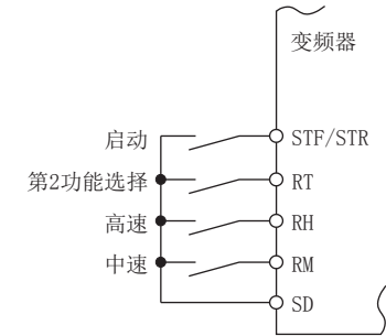
第 2 功能的接线图示例
