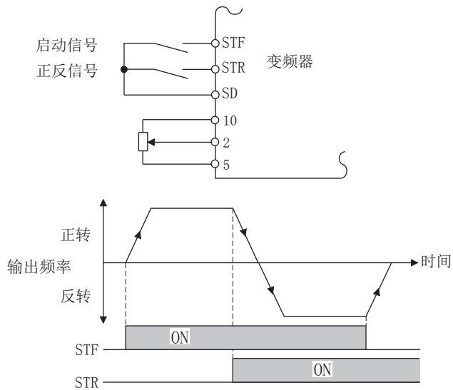
2 线式连接例（Pr. 250 = “8888”）
