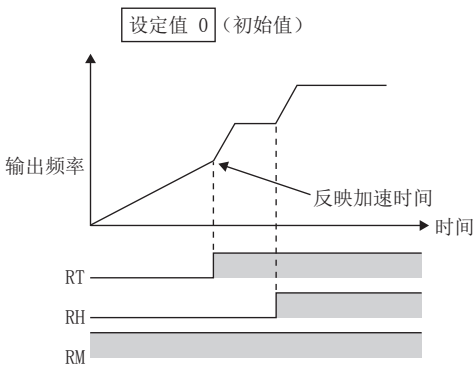
第 2 加减速时间示例
