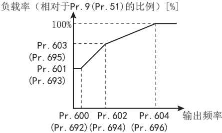
连续运行特性
