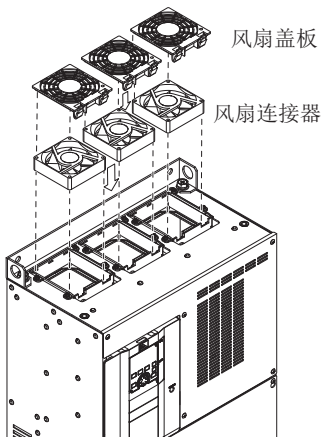
FR-A820-01870 (37K) 及以上 FR-A840-00930 (37K) ～ FR-A840-03610 (132K)
