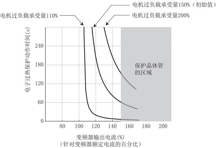
电机过负载承受量设定示例（设定Pr. 9=“变频器额定的100%”时）
