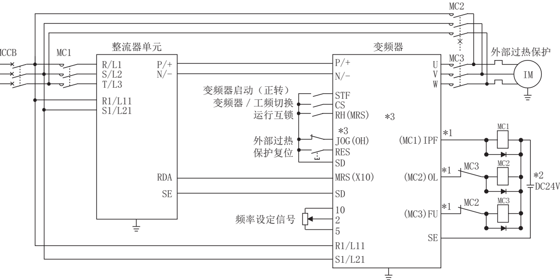
整流器分离类型
